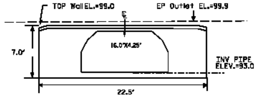
OUTLET
